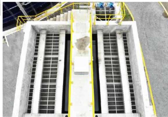
Lamella Clarifier for flow 2800 mcd in Mexico Clarificador de láminas para caudal 2800 mcd en México
