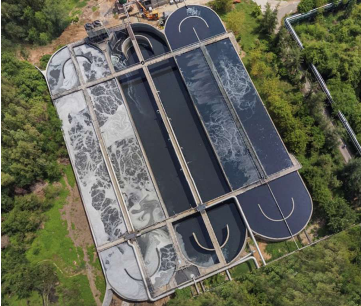
Aerial View for One of Worlds Largest Textile ZLD facility in India for flow 9000 mcd Vista aérea de una de las instalaciones ZLD textiles más grandes del mundo en India para un flujo de 9000 mcd
